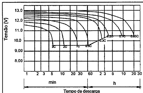
Característica de Descarga (25°C)
