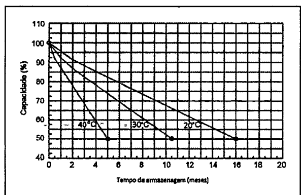
Característica de autodescarga (25°C)
