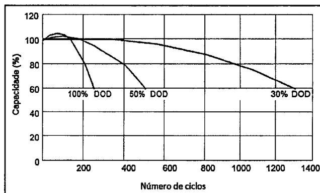
Nº Ciclos X Profundidade DOD (25°C)
