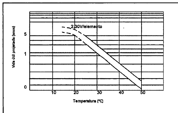
Vida útil em flutuação X Temperatura
