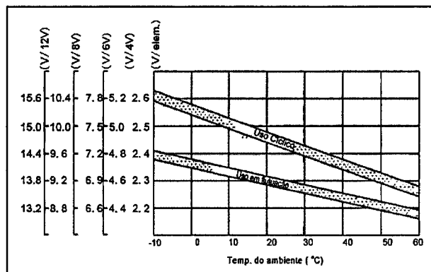
Tensão de Carga X Temperatura
