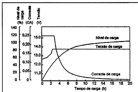
Característica de Carga (25°C)
